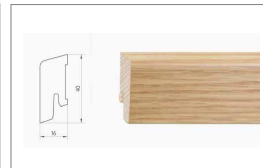
Abb. 8: Symbolfoto Sockelleiste
